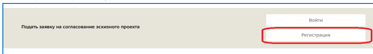
Рис. 1. Кнопка Регистрация
