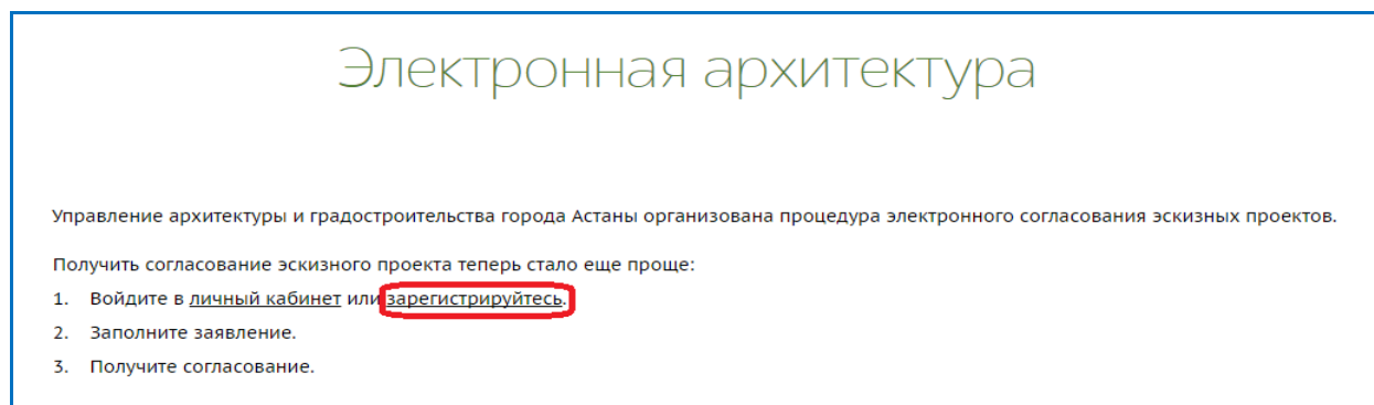
Рис. 2. Ссылка Зарегистрируйтесь
